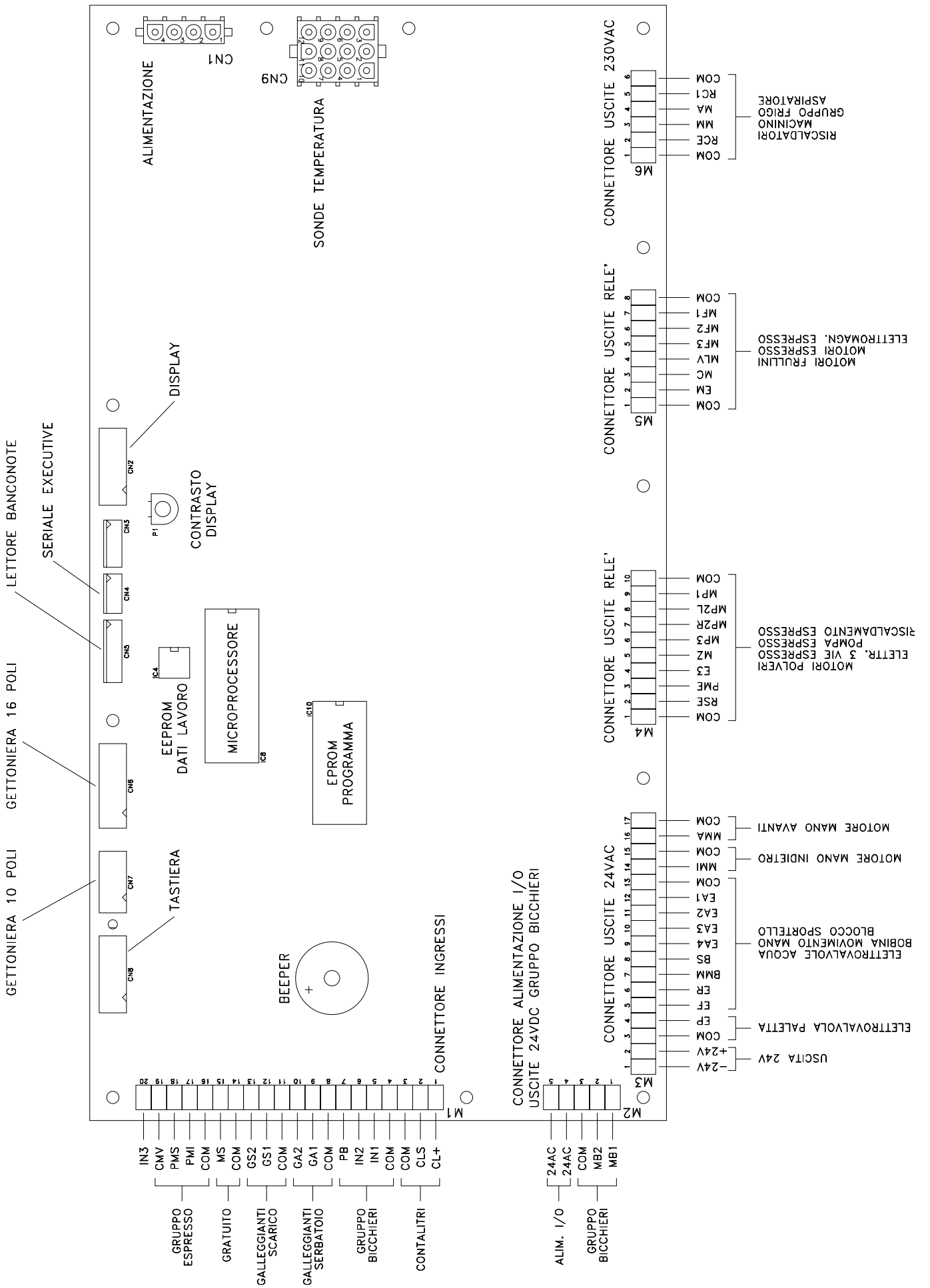
Layout della scheda DB8B e connessioni esterne
